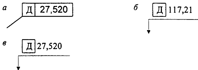
Рисунок 1 - Обозначение действительной отметки поверхности
