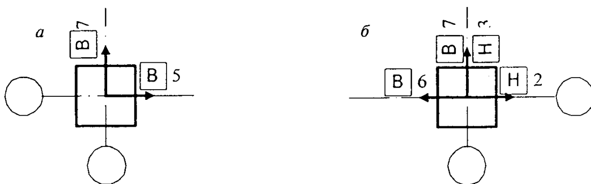
Рисунок 3 - Примеры указания действительных отклонений осей элементов от разбивочных осей на плане
