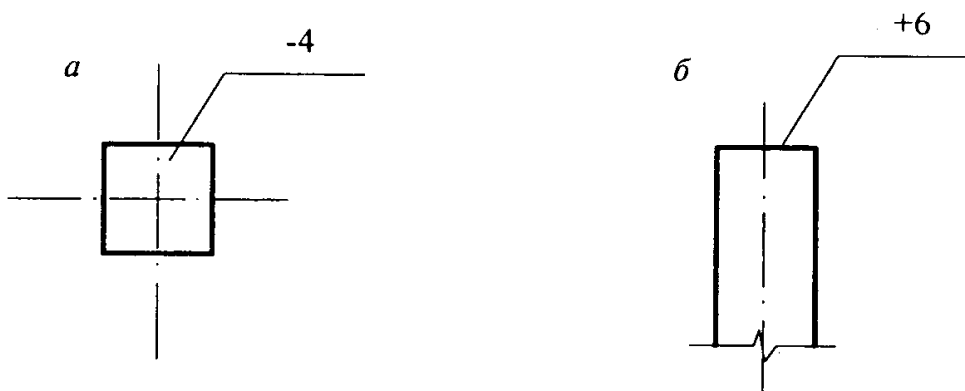
Рисунок 2 - Примеры указания действительных отклонений поверхностей
